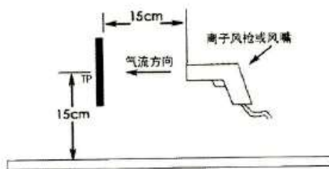
图 A.6 离子风枪/风嘴测试示意图
