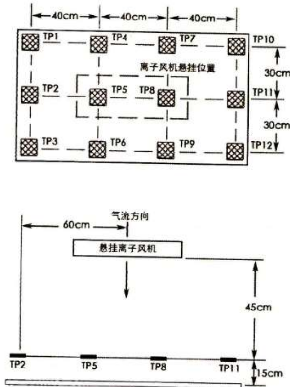
图 A.5 悬挂式离子风机测试正视剖面示意图
