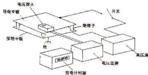
图 A.1 充电板监测仪结构示意图
