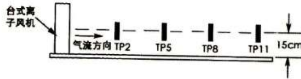
图 A.3 台式离子风机正视剖面示意图
