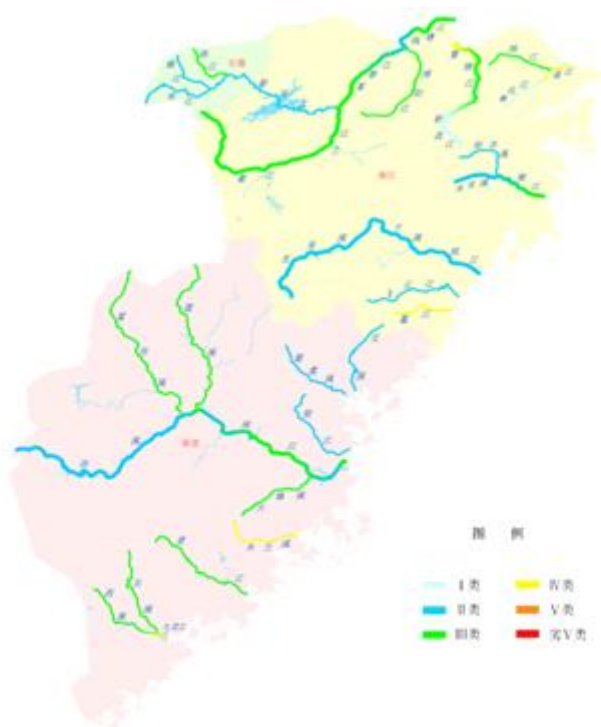
2013年浙闽片河流水质分布示意图
