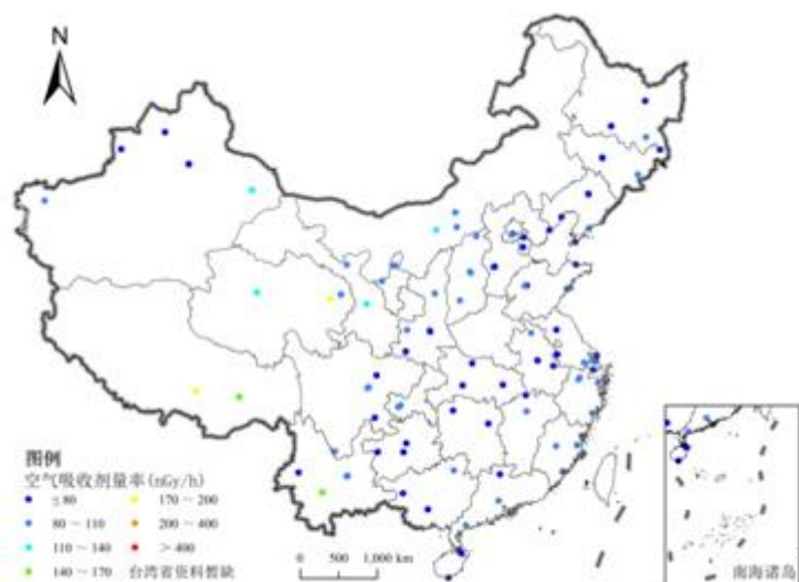
2013年全国辐射环境自动监测站实时连续 \gamma 辐射空气吸收剂量率分布示意图
