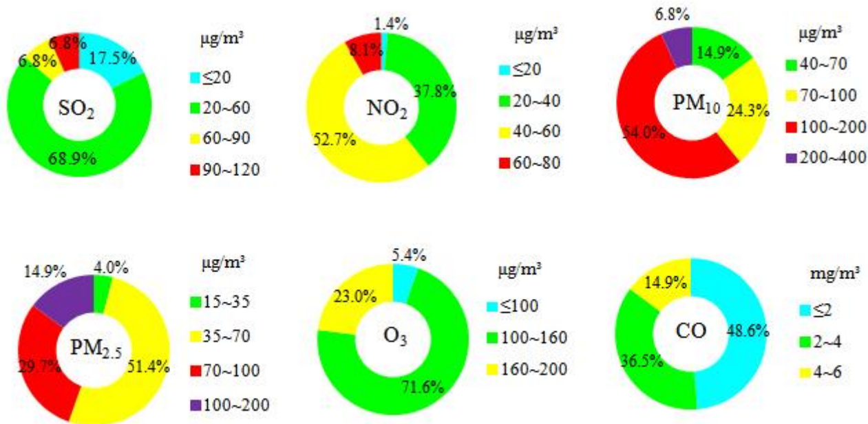
2013年新标准第一阶段监测实施城市各指标不同浓度区间城市比例
