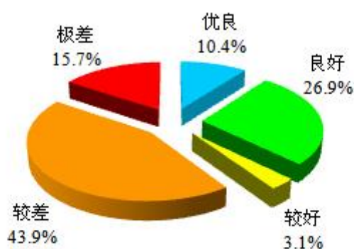
2013年地下水监测点水质状况
