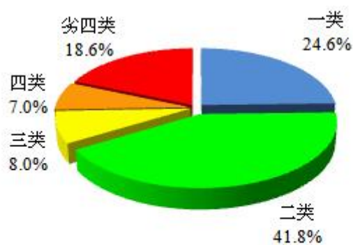
2013年全国近岸海域水质状况
