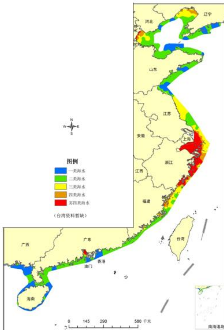
2013年全国近岸海域水质分布示意图
