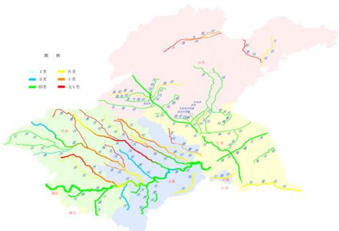
2013年淮河流域水质分布示意图
