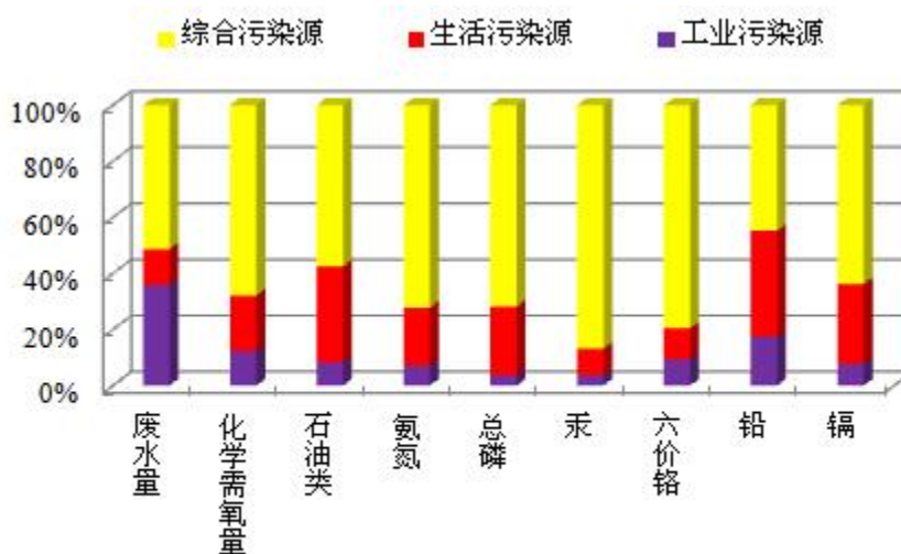
2013年不同类型直排海污染源主要污染物排放情况
