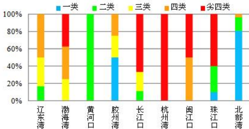
2013年重要海湾水质状况
