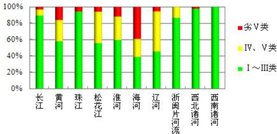
2013年十大流域水质状况
