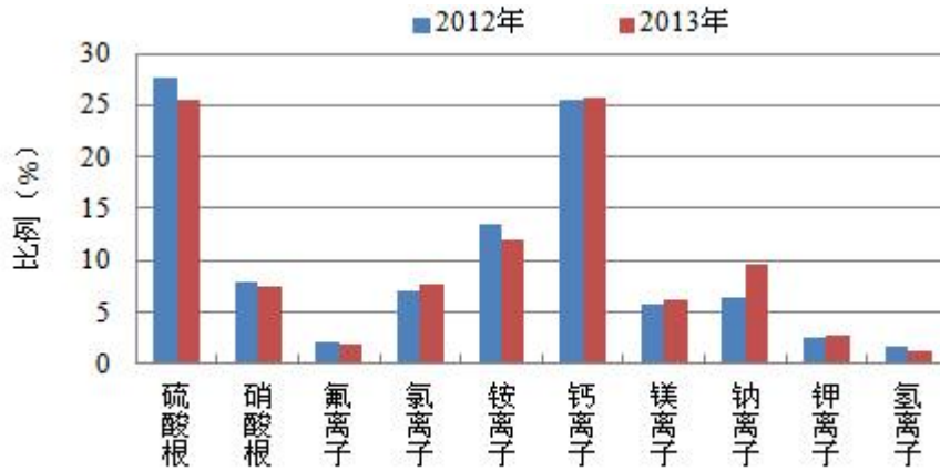
降水中主要离子当量浓度比年际变化
