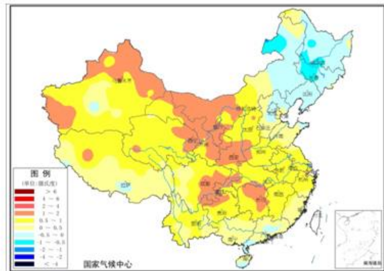
2013 年全国年平均气温距平分布示意图
