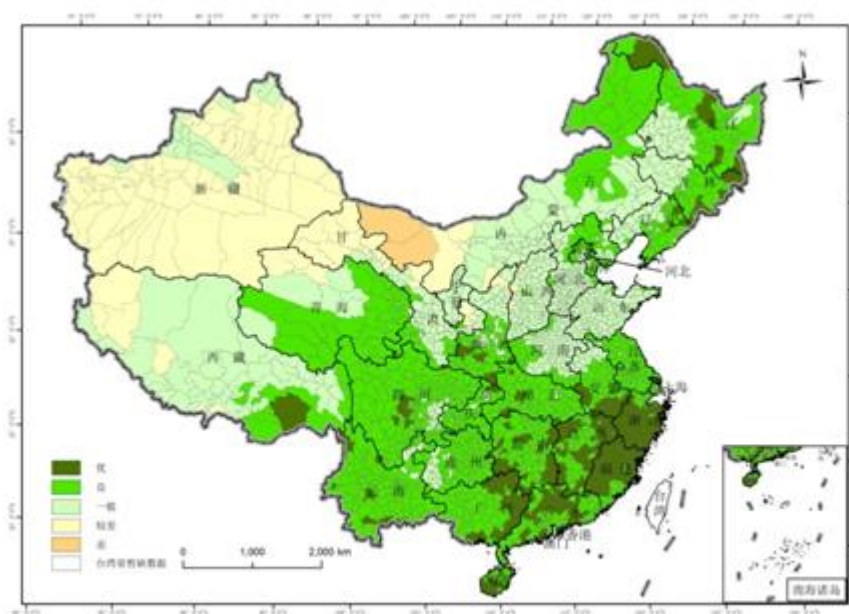
2012年全国县域生态环境质量分布示意图
