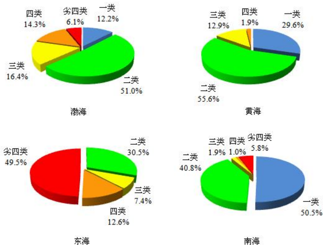
2013 年四大海区近岸海域水质状况
